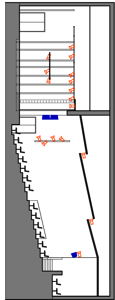
PODUZNI PRESEK
