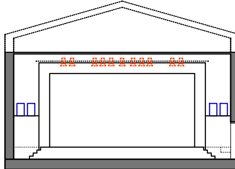
POPREČNI PRESEK - POGLED KA BINI
