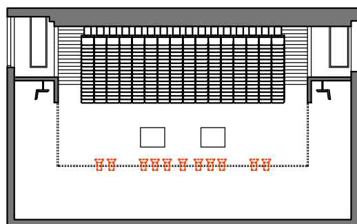
POPREČNI PRESEK - POGLED KA GLEDALISTU
